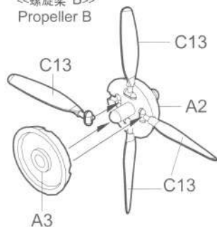
<<螺旋桨 B>> Propeller B
