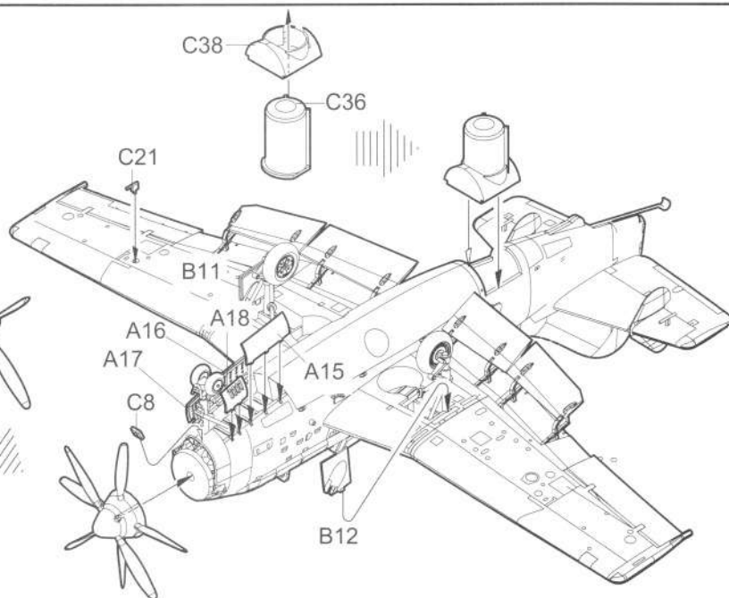
<<螺旋桨 A>> Propeller A
