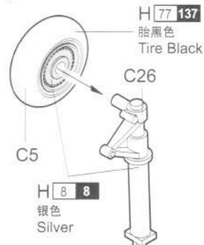
<<右侧主起落架>> Right main undercarriage
