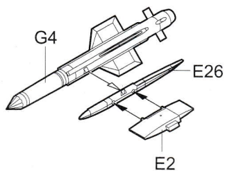
<<火光导弹-右侧>> Fire streak missile-R
