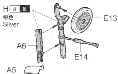
<<右侧主起落架>> Right main undercarriage
