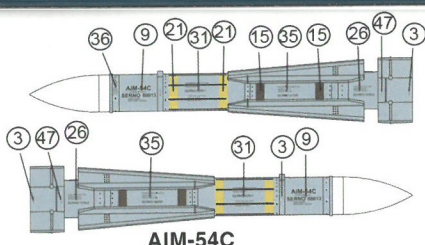
AIM-54C
