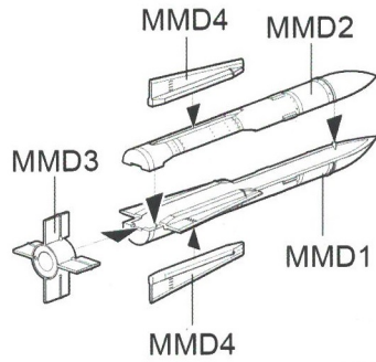
AIM-54C
