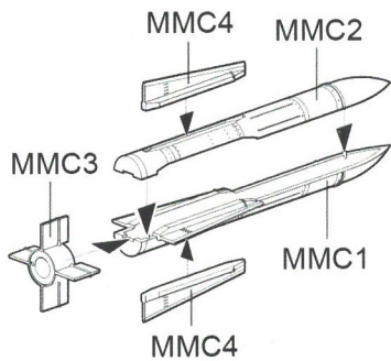
AIM-54A
