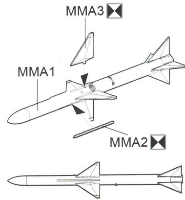
AIM-7E
