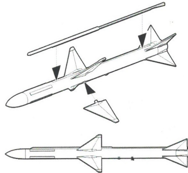
AIM-7M
