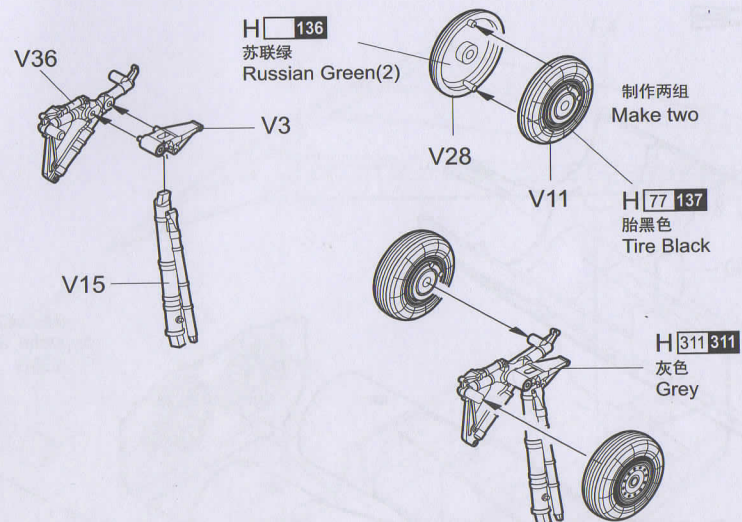
《左侧主起落架》 Left main undercarriage
