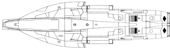
《上部机身》 Top Fuselage
