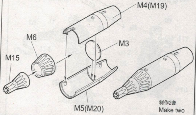
R3S 导弹 R-3S missiles
