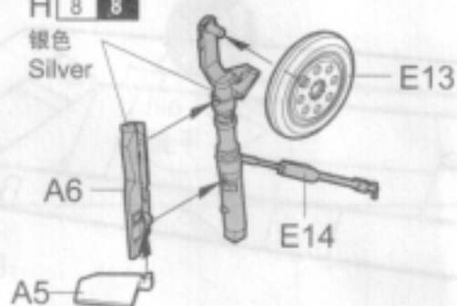
«右侧主起落架» Right main undercarriage
