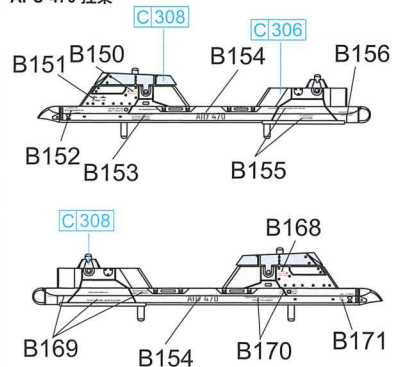
APU-470 Pylon APU-470 挂架
