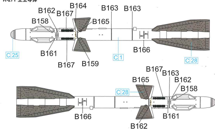
R-27T Missile R-27T 空空导弹
