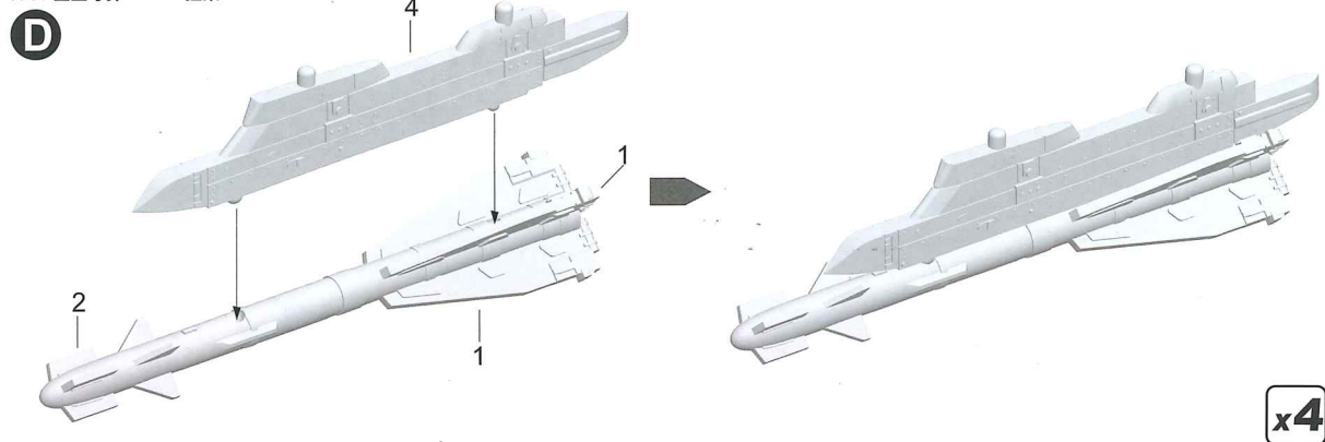
R-60 Missile + P-62 Pylon R-60 空空导弹 + P-62 挂架
