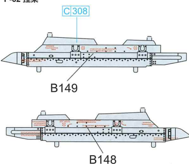
P-62 Pylon P-62 挂架
