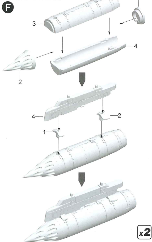
PTB-1150 Tank + PTB-1150 Pylon PTB-1150 油箱 + PTB-1150 挂架
