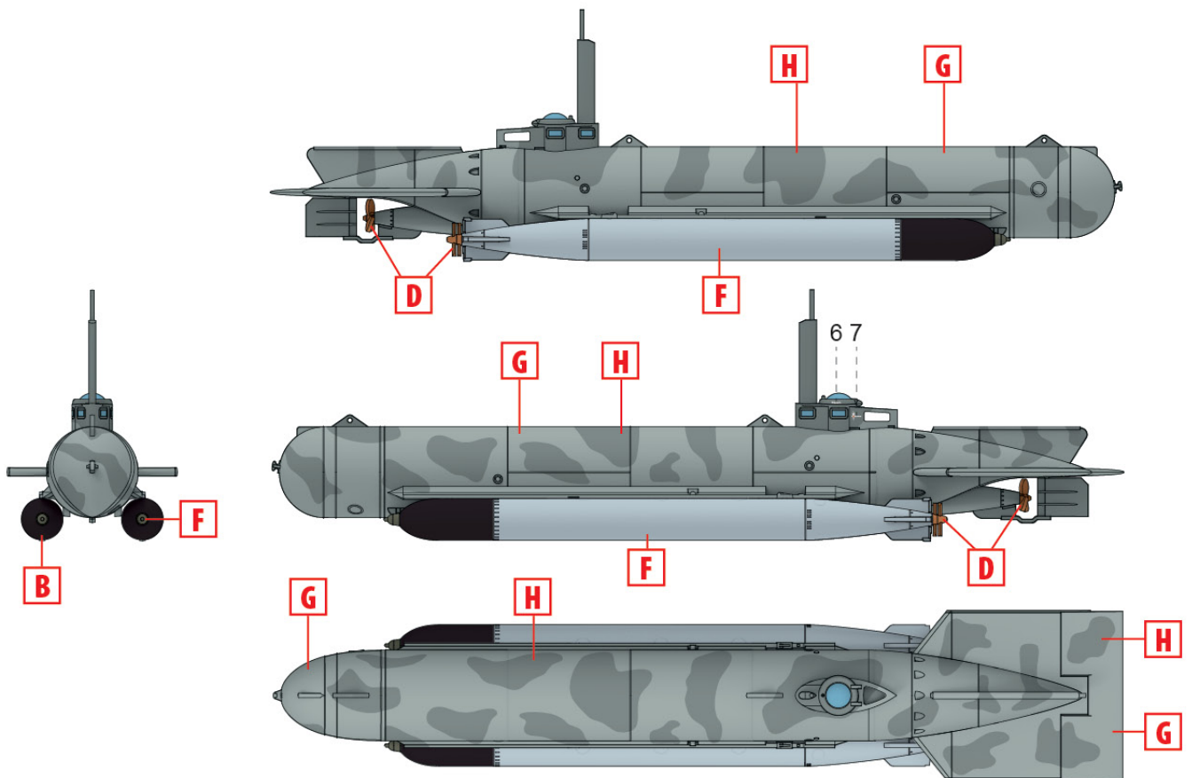
2) Міні-субмарина «Molch», з'єднання «К» (K-Verbände), Північне море, 1945 рік Midget submarine "Molch", formation "K" (K-Verbände), North Sea, 1945
