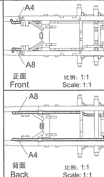
车架 Chassis
