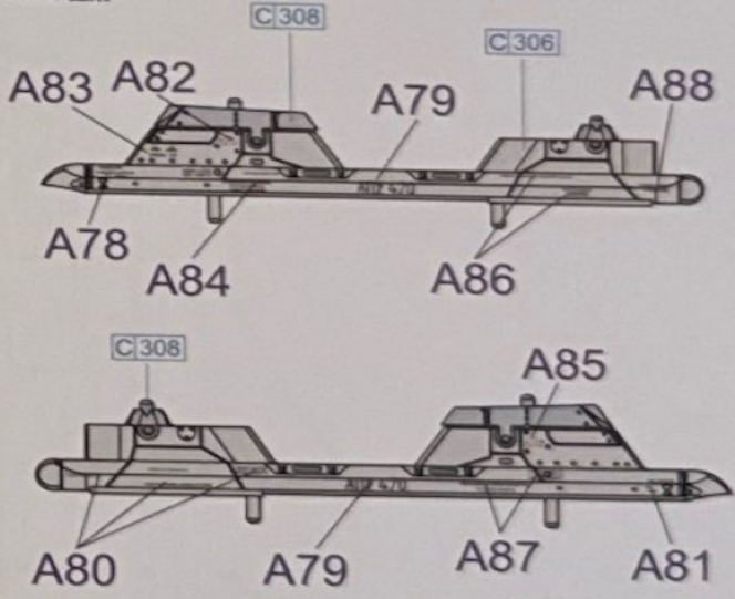
PTB-1500 Fuel Tank PTB-1500 副油箱
