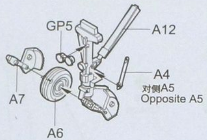
<<前起落架>> Nose undercarriage
