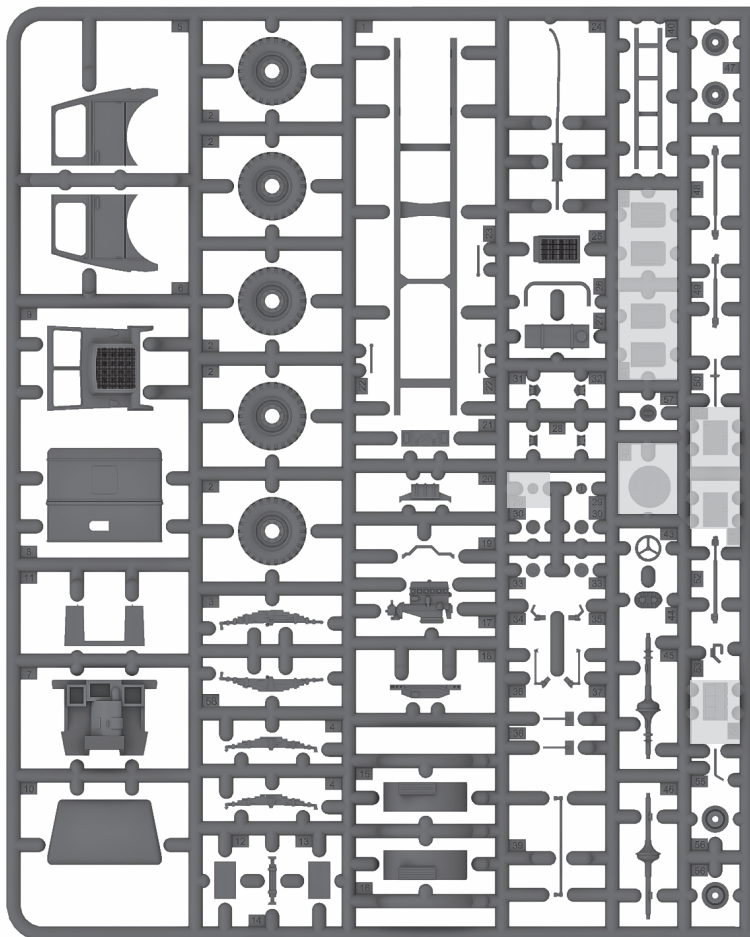
Ramka bez oznaczenia literowego / Frame with no letter
