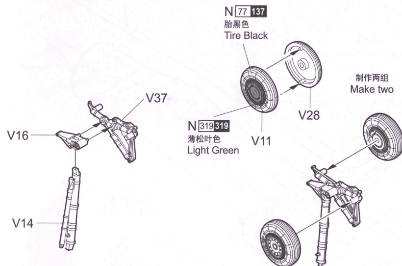
《右侧主起落架》 Right main undercarriage
