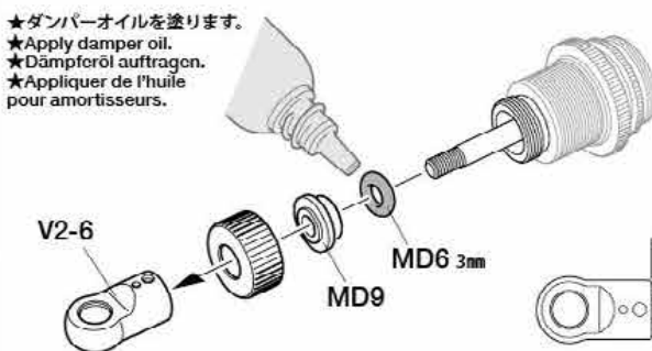
ロッドガイドキャップ Rod guide cap Kappe an der Gestängeführung Coupelle de guidage d'axe
