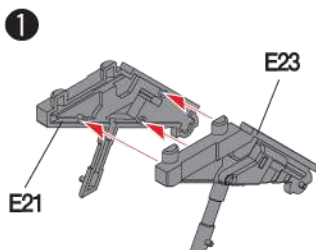
Lending gear 3 왼쪽 렌딩기어 3
